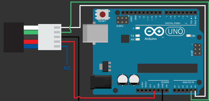
Arduino Uno
